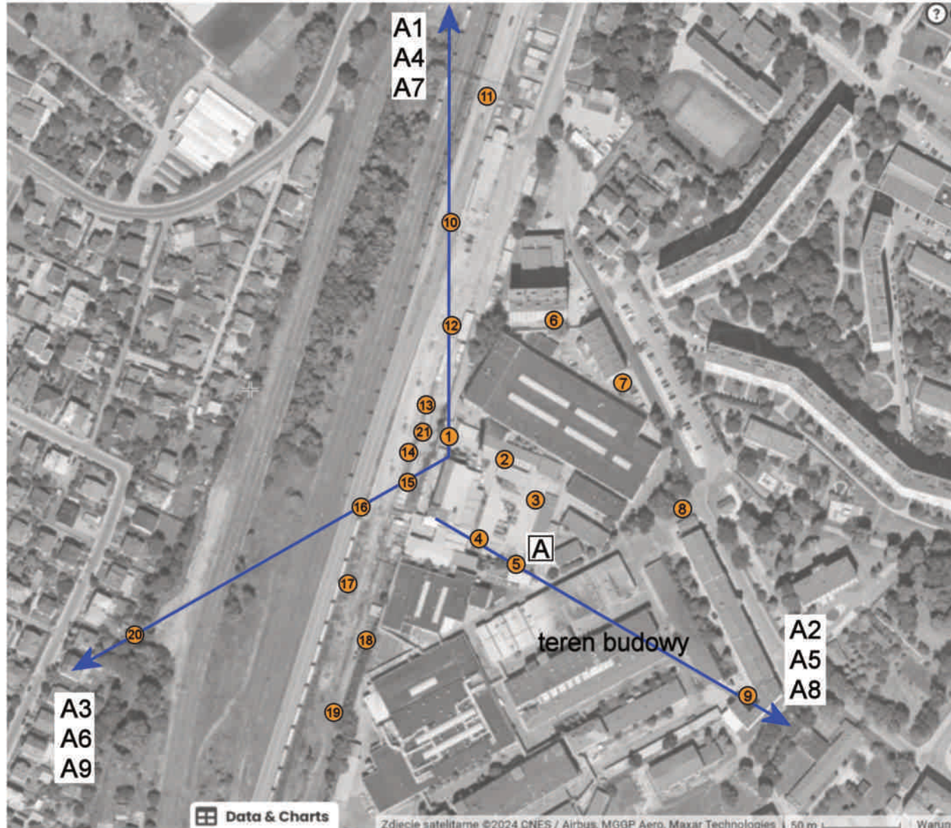
Azymuty anten P4
